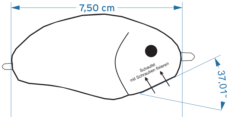
Draufsicht Form
